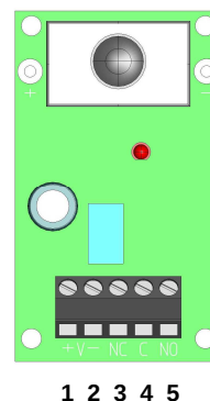
Fig. 1A (RX)
