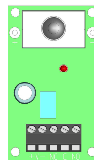
Fig. 1A (RX)
