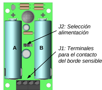
Fig. 1B (TX)
