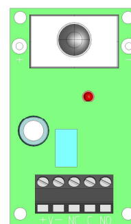
Fig. 1A (RX)
